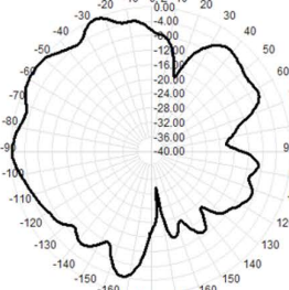
5650.0MHz Total(E2-YZ), Max= -0.49dB
