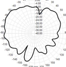
5450.0MHz Total(E2-YZ), Max= -0.35dB
