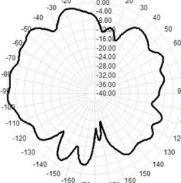
5850.0MHz Total(E2-YZ), Max= -0.90dB
