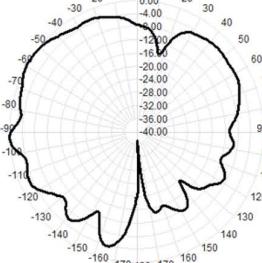
5550.0MHz Total(E2-YZ), Max= -0.52dB
