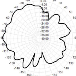
5950.0MHz Total(E2-YZ), Max= -0.22dB
