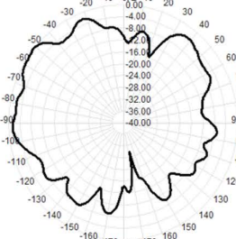
5750.0MHz Total(E2-YZ), Max= 0.33dB
