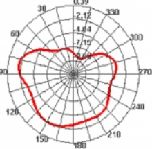
880.000MHz E1
