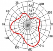
880.000MHz H
