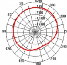
884.000MHz H
