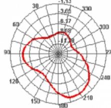
698.000MHz E2
