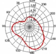
715.800MHz E2
